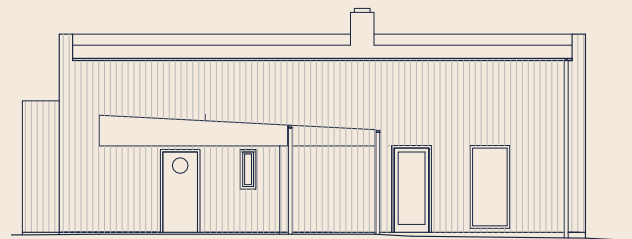
SEKTION F-F
